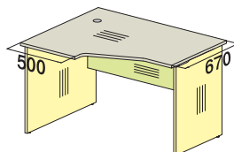
изоб. 76S053 зерк. 76S054 1180x950x737
