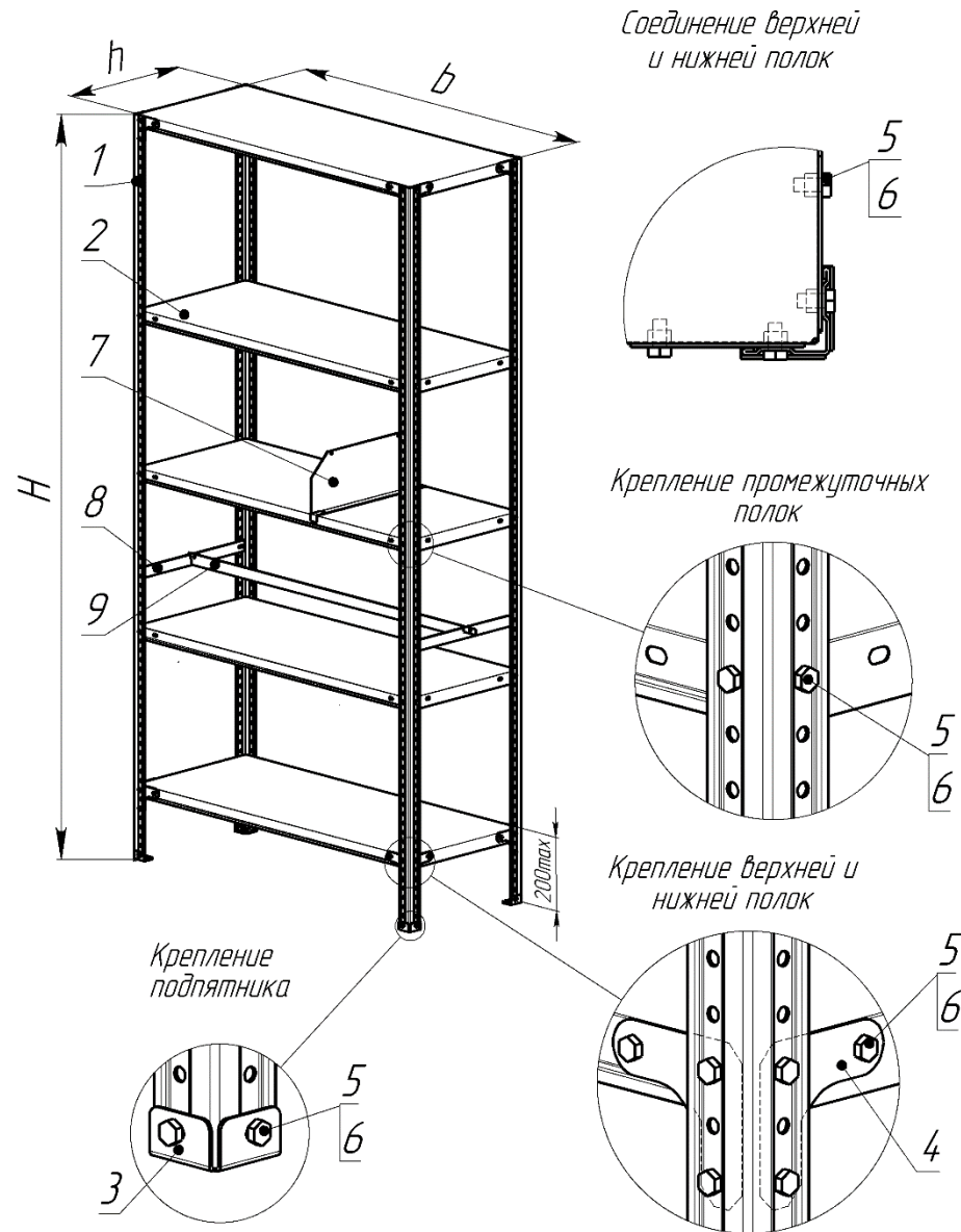
Рис. 1 – Схема сборки стеллажа
